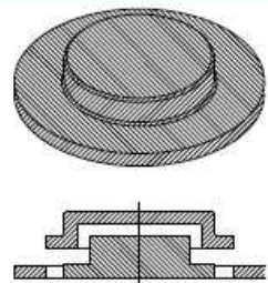
RIFILATURA PARTICOLARI IMBUTITI TRIMMING OF DRAWN PIECES TIEFZIEHEN SCHNITT
