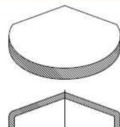
TAGLIO E BORDATURA FONDI CONICI TRIMMING AND FLANGING OF CONICAL BOTTOMS SCHNEIDEN UND BORDELN KONISCHER BODEN
