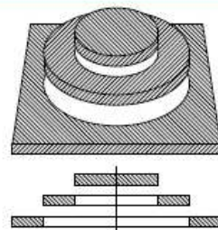
TAGLIO ANELLI - RING TRIMMING - SCHEIBRINGSCHNITT
