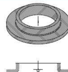
FLANGIATURA INTERNA ANELLI RING INSIDE FLANGING SCHEIBRINGBORDELN
